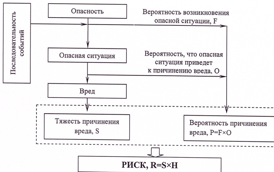
Рисунок 1 – Графическое представление соотношения между опасностью, последовательностью событий, опасной ситуацией и вредом
